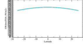
rsdtzon
