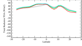
rttzon
