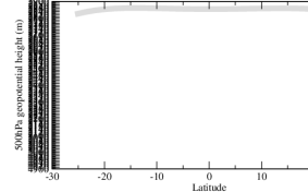
zg500zon
