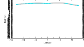
sstzon
