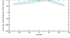
rttczon
