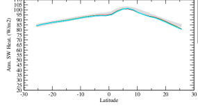
rsahzon
