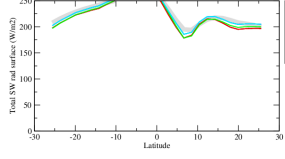
rstczon
