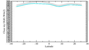
rlutczon
