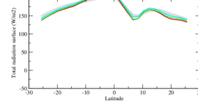
rtszon
