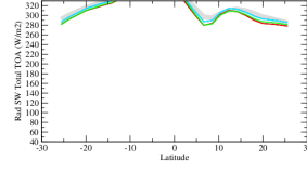
rsttczon
