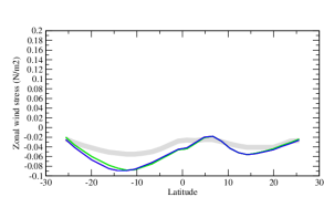
tauzon
