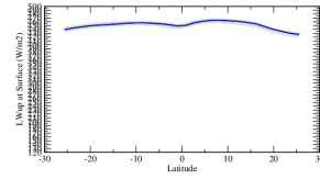
rluszon
