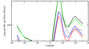
rsutzon
