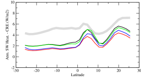
rsahcrezon
