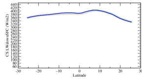
rldscszon
