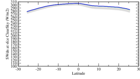
rsdscszon
