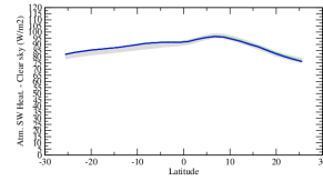
rsahcszon
