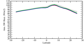
rsahzon
