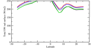
rstszon
