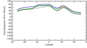
rttzon
