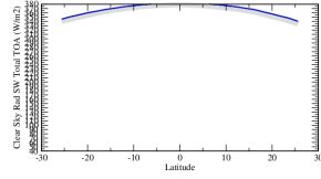
rsttcson
