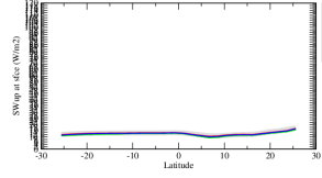
rsuzon
