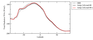
rttczn
