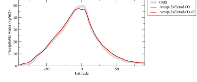
prwzon
