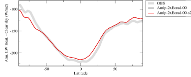
ralhcszon
