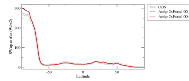
rsuzcn
