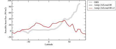
hflsszon
