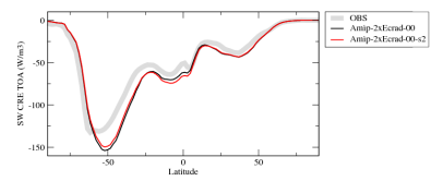
creltzon
