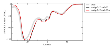
crelson
