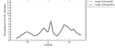
procezon
