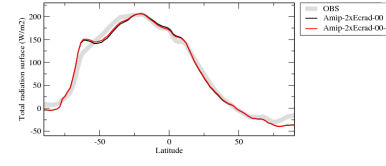
rtsczn
