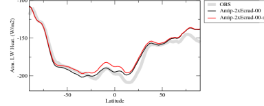
ralhzon
