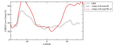
chlzon
