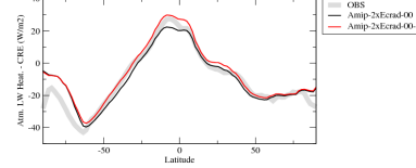
ralhcrezon
