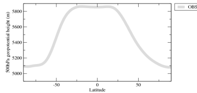
zg500zn
