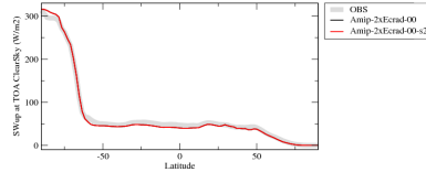
rsutsczn
