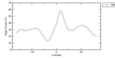
chlcalipsozon
