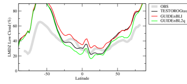
chlzon
