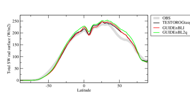
rstszon
