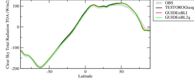
rttczn
