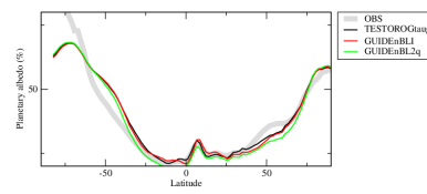
albtzon
