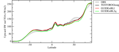
rsutzcn
