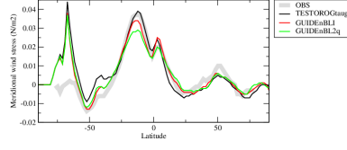
tauvzn
