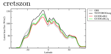
hflszon
