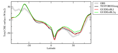
cretzon
