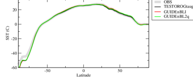
sstzn
