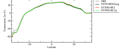
taszn
