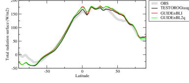
rtsczn
