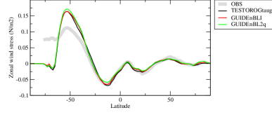
tauzzn
