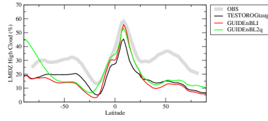
chlhzon
