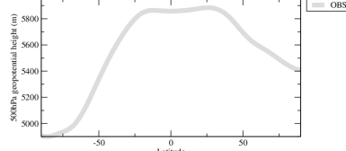
zg500zn
