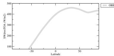
rsdtzon
