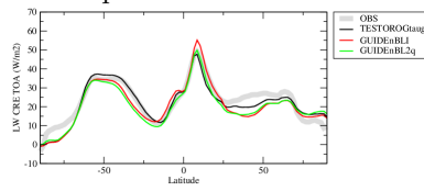
crelcalipsozon
