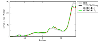
rsuzcn
